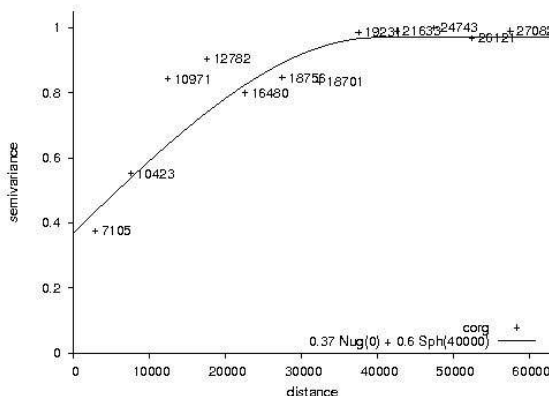
Abb. 2: Omnidirectionales Semivariogramm für organischen Kohlenstoff im Oberboden unter Ackerland.
